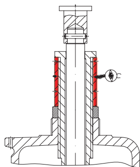
自锁衬套
