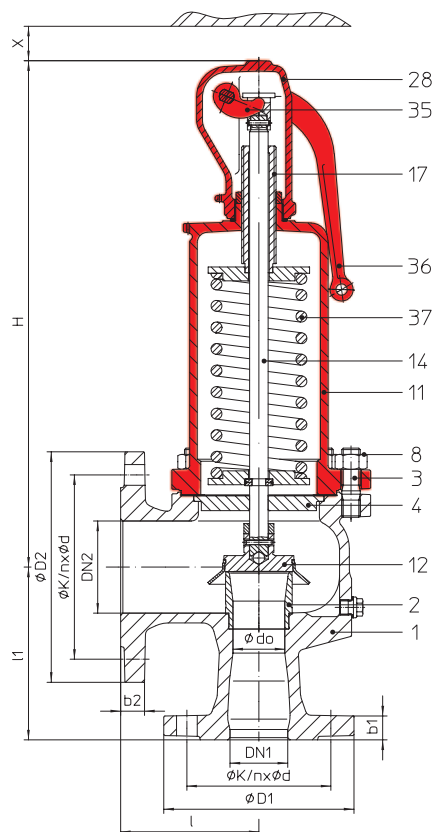
Fig. ...901型 闭式阀帽 闭式顶盖 带手柄
