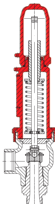
Fig. 25.943 气密式顶盖,不带手柄
