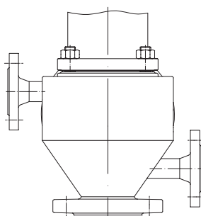
加热夹套
