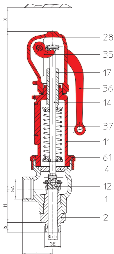
Fig. 25.941 闭式顶盖,带手柄
