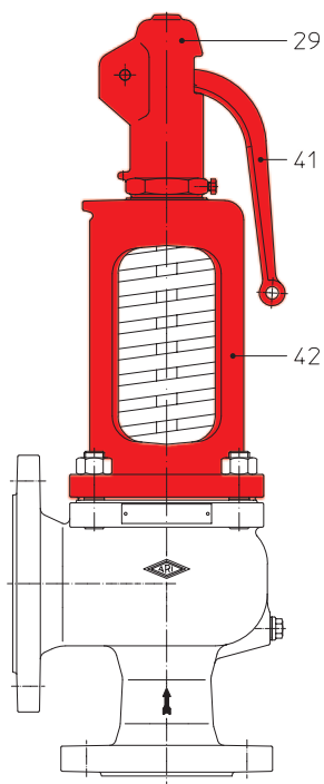
Fig. ...902型 开式阀帽 开式顶盖 带手柄
